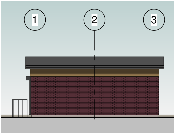
4 South 1 : 100
